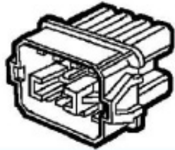
Can connector PartNo: 41 17 461 Pin partNo: 41 150 77
